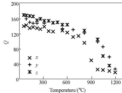
图 3 2.0 GPa 下斜长角闪岩的 Q 值-温度曲线 Fig. 3 Q versus temperature in amphibolite at 2.0 GPa
