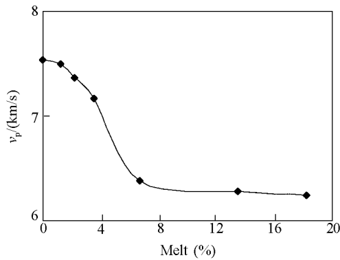
图 4 2.0 GPa 下斜长角闪岩的 v_p -Melt 曲线 Fig. 4 v_p versus Melt in amphibolite at 2.0 GPa
