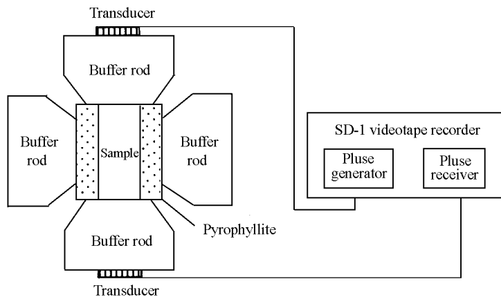
图 1 弹性波速度及其衰减的实验装置示意图
