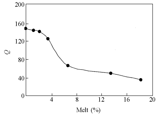
图 5 2.0 GPa 下斜长角闪岩的 Q-Melt 曲线 Fig. 5 Q versus Melt in amphibolite at 2.0 GPa
