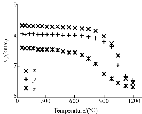
图 2 2.0 GPa 下斜长角闪岩的 v_p -温度曲线 Fig. 2 v_p versus temperature in amphibolite at 2.0 GPa
